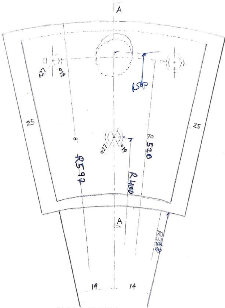
SECTION-A
